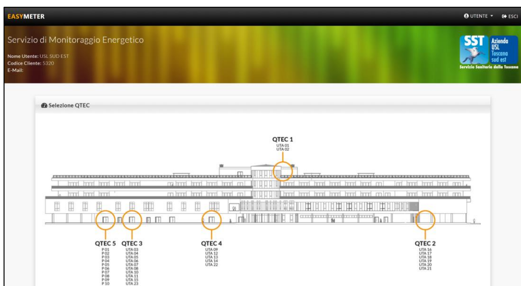
Figura 10. Piattaforma di monitoraggio delle UTA e delle elettropompe Ospedale Grosseto, Azienda USL Toscana Sud Est
